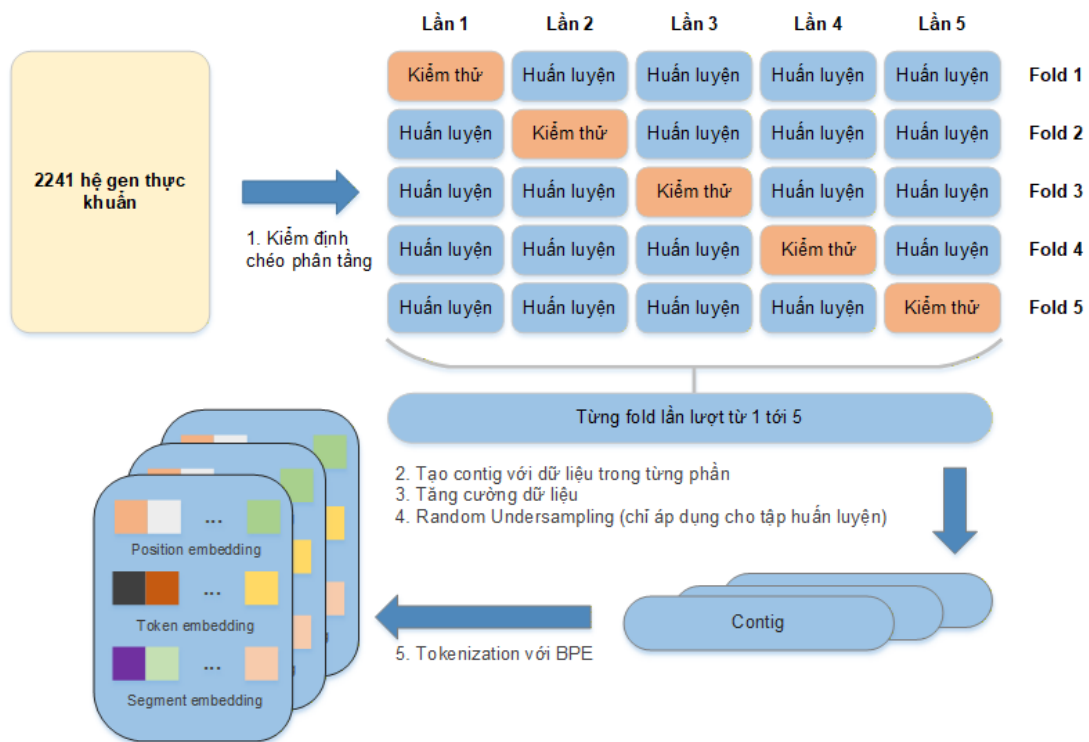
Hình 3.1: Pipeline tiền xử lý năm bước: chia dữ liệu ở mức hệ gen (5-fold phân tầng), tạo contig bằng cửa sổ trượt, tăng cường dữ liệu bằng chuỗi bổ sung đảo ngược, cân bằng lớp bằng lấy mẫu giảm ngẫu nhiên chỉ trên tập huấn luyện và mã hóa BPE
