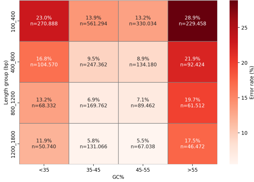
Hình 4.3: Bản đồ nhiệt tỉ lệ lỗi của PhaBERT theo lưới hai chiều nhóm độ dài \times khoảng GC (số liệu gộp trên tập kiểm định năm phần)
