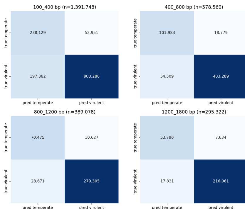
Hình 4.2: Ma trận nhầm lẫn của PhaBERT trên bốn nhóm độ dài contig (số liệu gộp trên tập kiểm định năm phần)
